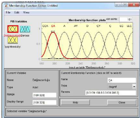
Şəkil 5. Dalğa uzunluğu üçün qeyri-səlis üzv funksiyalarının redaktə pəncərəsi
