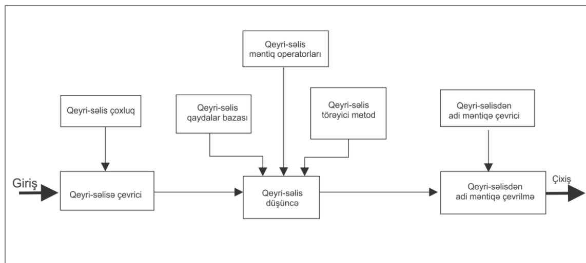
Düz metodlar iki kateqoriyaya bölünür: Mamdaninin Düz Metodu və Takaqi-Suqeno-Kanqın (TSK) qeyri-səlis modelləşməsi. Takaqi-Suqeno-Kanq metodu 1985-ci ildə [16] təklif olunmuşdu, o Mamdani metoduna çox oxşayır: törəyici prosesi oxşardır, giriş verilənləri fəzzifikasiyası və qeyri-səlis operatorun tətbiqi eynilədir. Mamdani və Suqeno metodlarının bir-birindən əsas fərqi ondan ibarətdir ki, Suqeno metodunun çıxış üzv funksiyaları ya xəttidir, ya da ki sabit. Suqeno metodu ilə ərsəyə gələn sistem Mamdani sisteminə nəzərən daha kompakt və hesablanma üçün effektiv tərzə malik olduğundan, o qaçılmaz olaraq qeyri-səlis modellərin quruluşunda adaptiv texnikalardan istifadəni sağlar. Bu adaptiv texnikalar üzv funksiyalarını ayarlamaq üçün istifadə edilir ki, qeyri-səlis sistem verilənləri daha dürtüst modelləsin.
