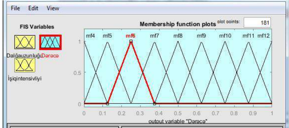
Şəkil 6. Rəng dərəcəsi üçün qeyri-səlis üzv funksiyalarının redaktə pəncərəsi
