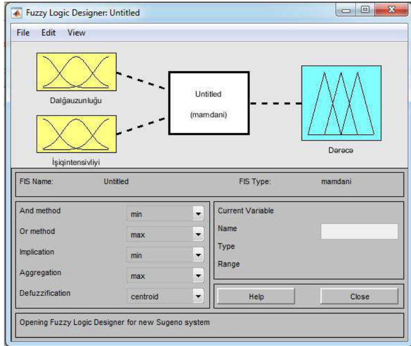
Şəkil 4. Rəng Tanınma sistemi üçün Üzv Funksiyalarının redaktə pəncərəsi
